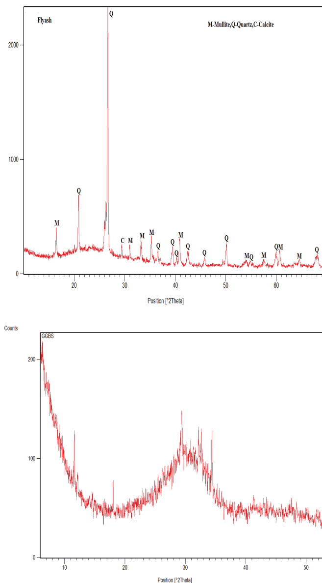
Rys. 3. Dyfraktogramy popiołu lotnego (u góry) i żużla wielkopieczowego (na dole)
